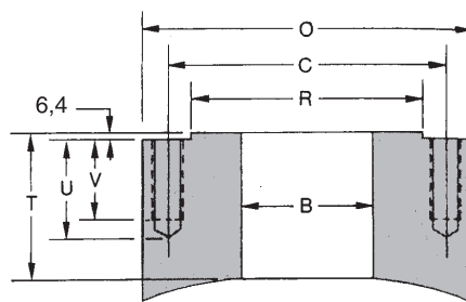
MONTAGGIO DI TESTA HEAD MOUNT
