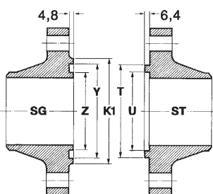
INCAMERATURA DOPPIA STRETTA SMALL TONGUE AND GROOVE
