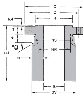
Connezioni rinforzate Reinforced connection "V 1 "
